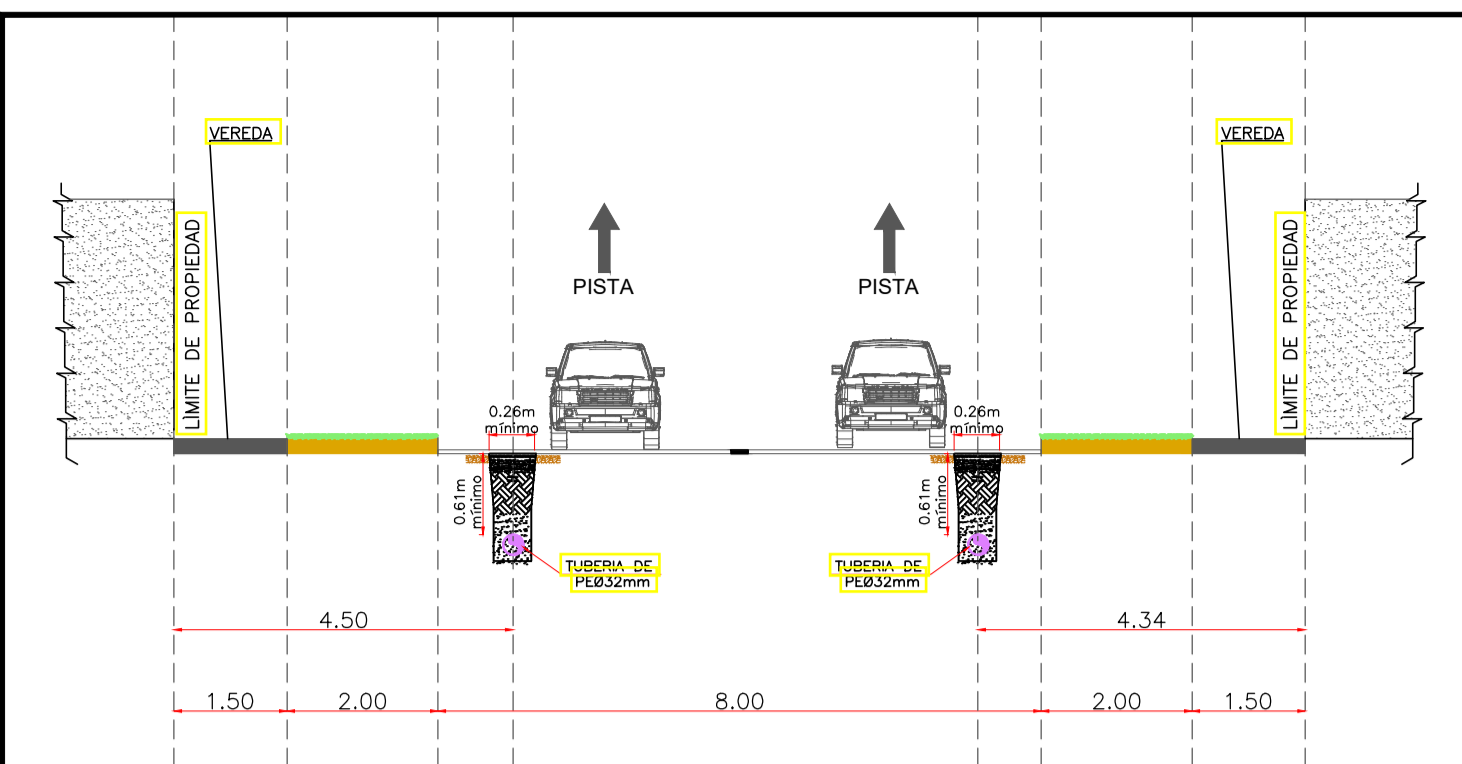
CORTE E-E CA JOSE DE RIVADENEYRA ALT. CA S/N(01) SC : 1/100
