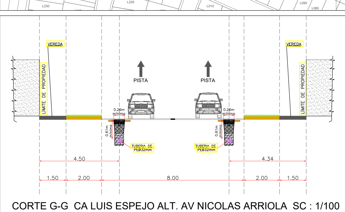
CORTE G-G CA LUIS ESPEJO ALT. AV NICOLAS ARRIOLA SC : 1/100
