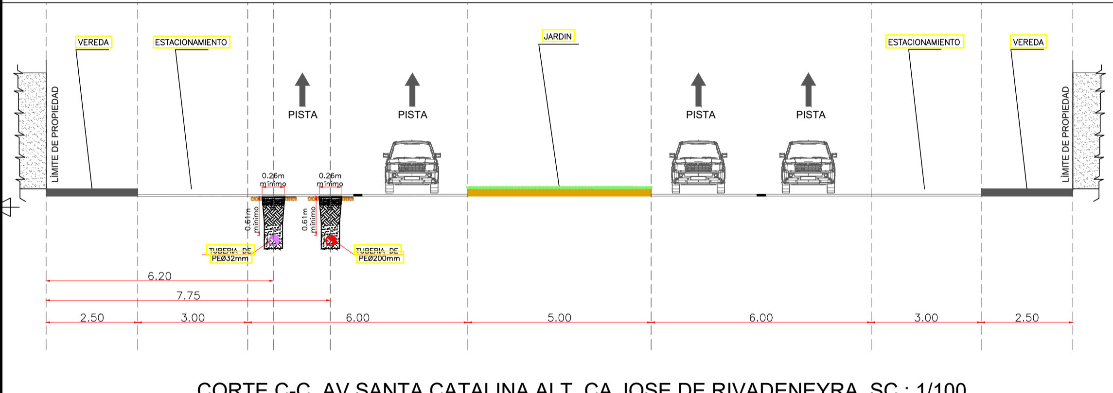
CORTE C-C AV SANTA CATALINA ALT. CA JOSE DE RIVADENEYRA SC : 1/100
