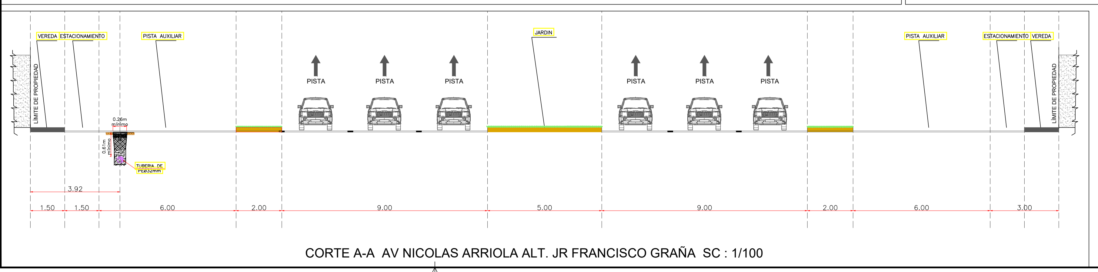
CORTE A-A AV NICOLAS ARRIOLA ALT. JR FRANCISCO GRAÑA SC : 1/100
