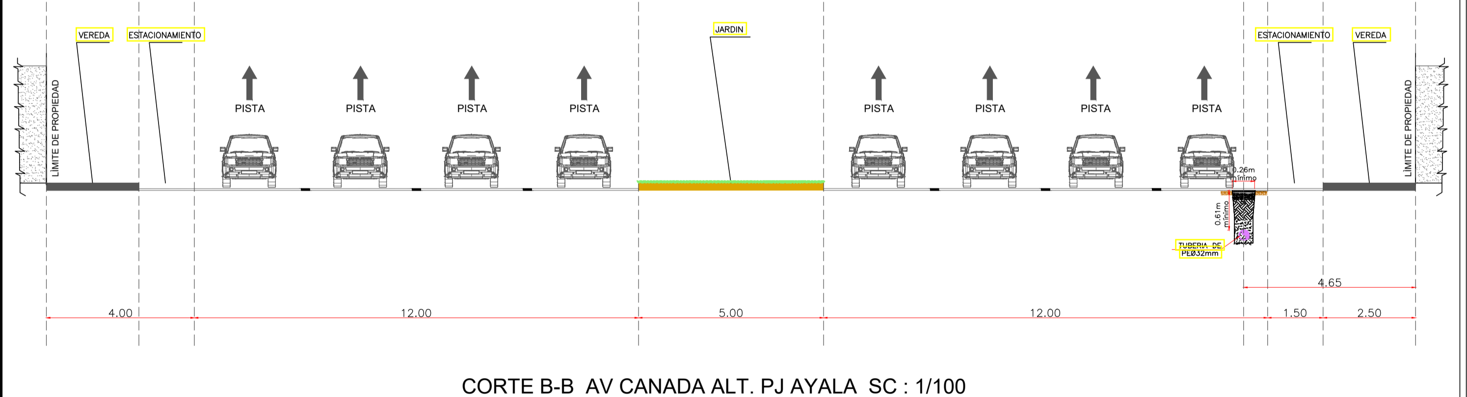
CORTE B-B AV CANADA ALT. PJ AYALA SC : 1/100
