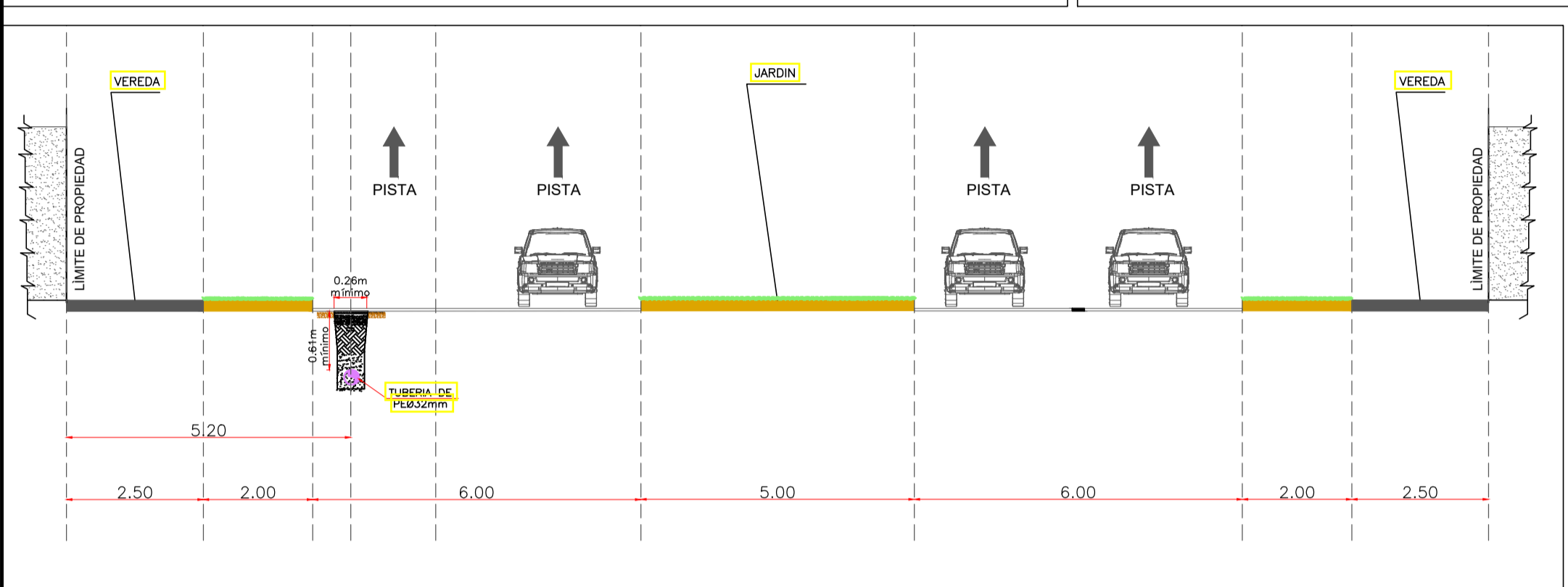
CORTE D-D AV SAN EUGENIO ALT. PJ RONCAL SC : 1/100
