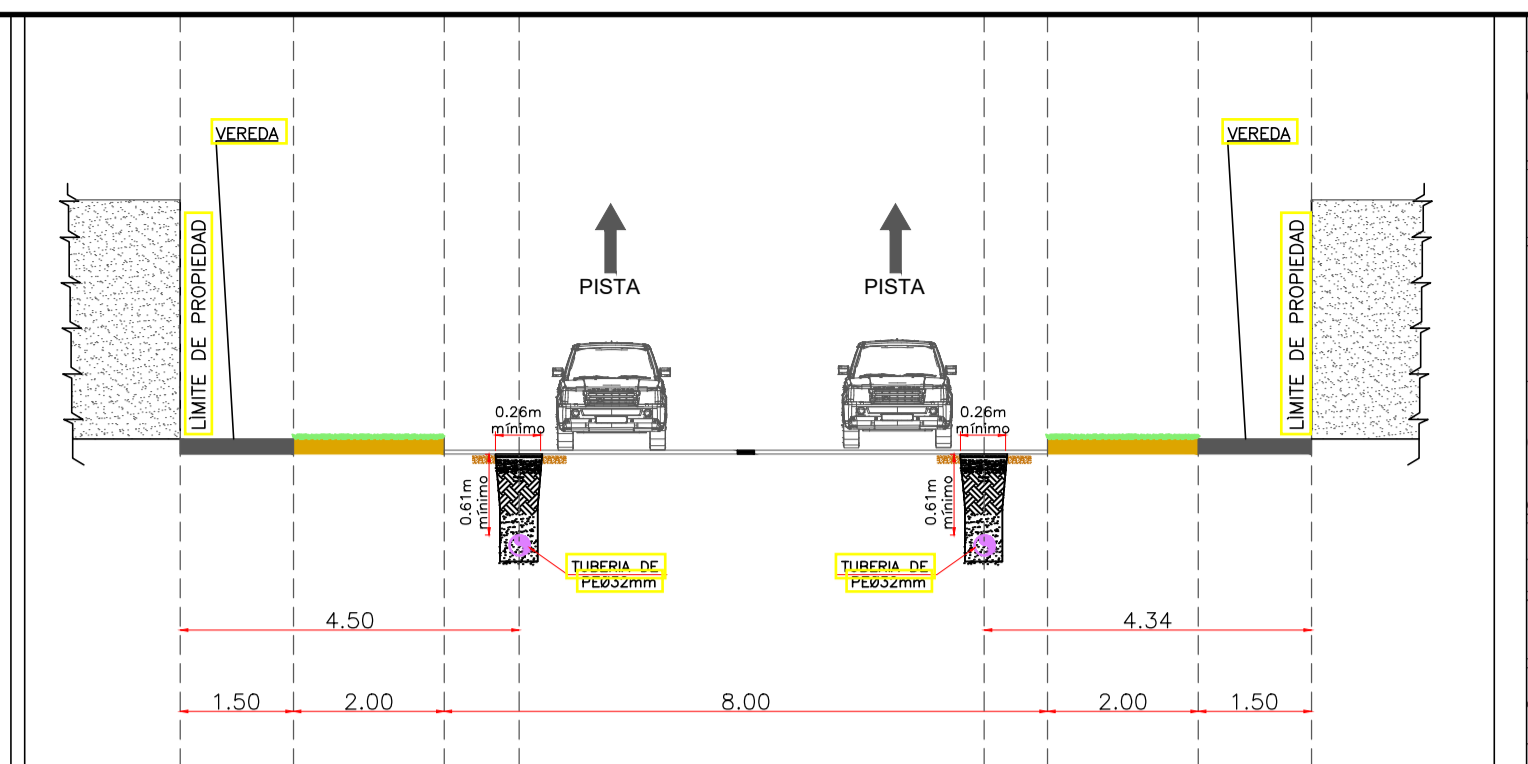
CORTE F-F CA MARIANO PACHECO ALT. CA MANZANARES SC : 1/100
